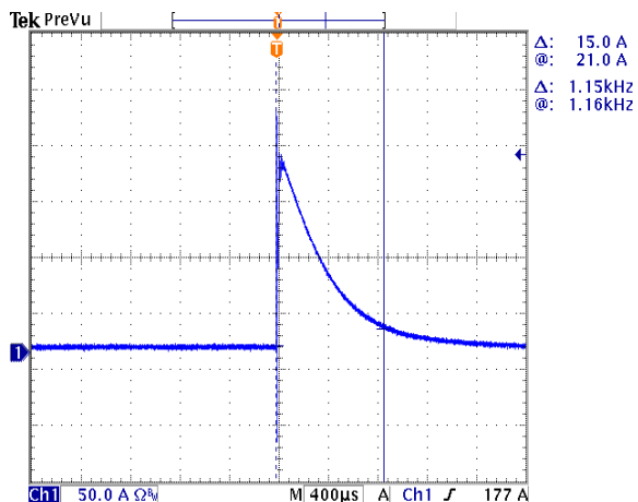
ESD-600S170DV( I_o=1700mA )
