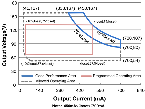
EUK-075S175DT(TT)
