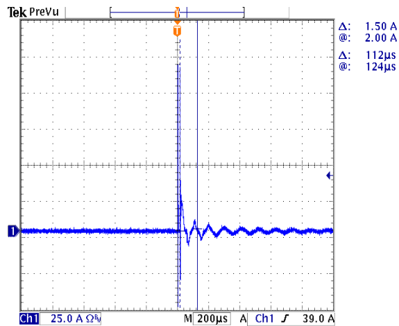
EUK-075S070DT(TT)(Io=700mA)
