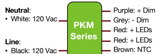
Wiring Diagrams
