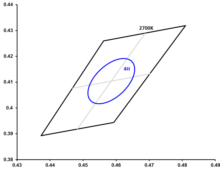
2700K 4Step
