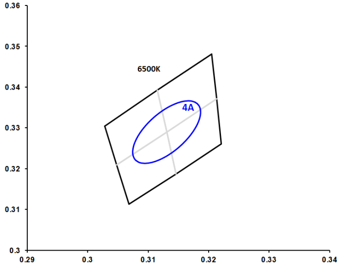
6500K 4Step
