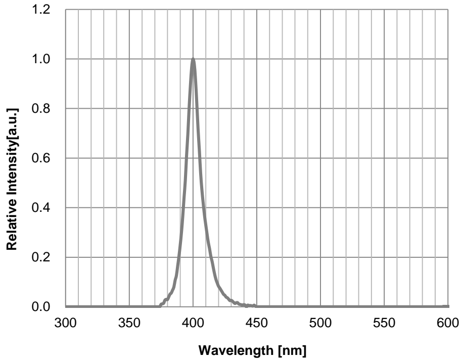
Fig 1. Spectrum, T_a=25^\circ\text{C} , I_F=180\text{mA}
